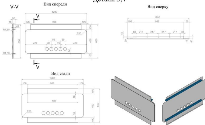
Лист 7 Детали 3,4
