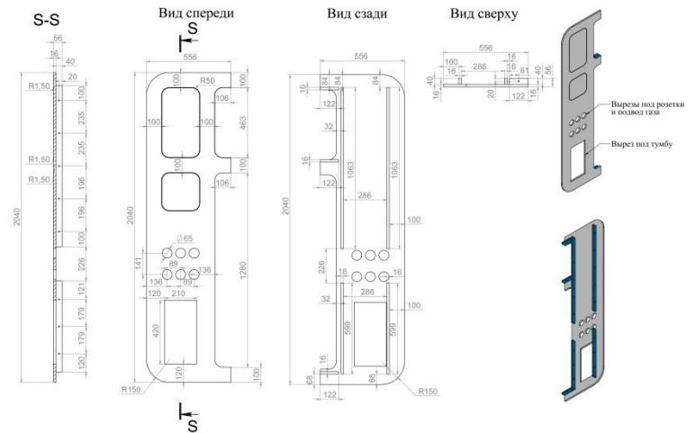
Лист 6 Детали 1,2
