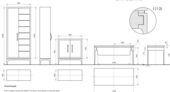
Фрагмент-разрез М 1:2
