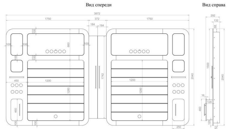
Лист 5.1 Общие размеры
