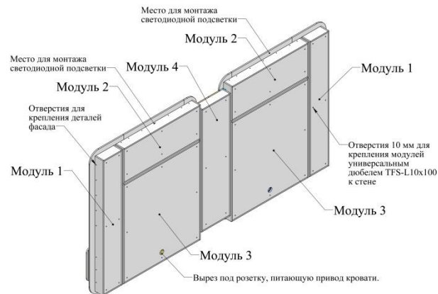
Лист 2.3 Обозначение деталей (ламинированный ДСП 16 мм) (модули для непосредственного крепления на стену)
