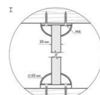
Фронт-разрез М 1:1
