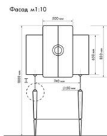
Проекция шкафа М1:10
